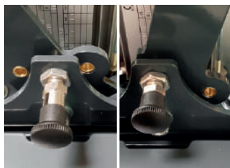
Dispositif de verrouillage avec goupilles d'arrêt (accessoires optionnels)
